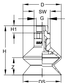
HSE43 External thread(egg)
